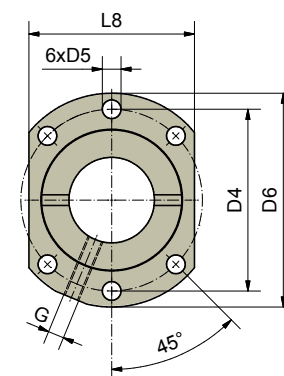
Hole pattern 1 to DIN 69051
